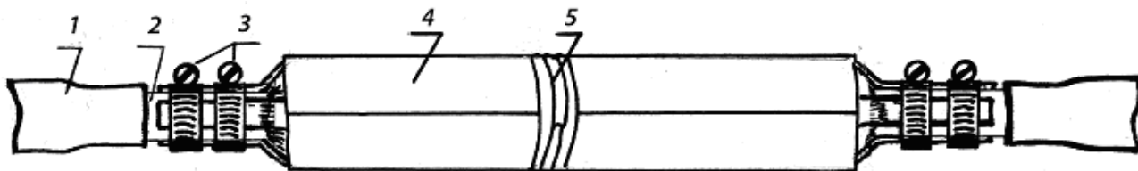
Рис. 4. Наложение каркаса на алюминиевые пластины: 1 – ТУТ продольной герметизации; 2 – алюминиевая оболочка; 3 – хомуты; 4 – каркас; 5 – бандаж из изолянты ПВХ.
