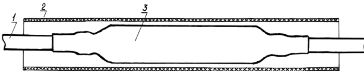
Рис. 6. Усадка наружной трубки ТУТ. Наружная трубка ТУТ должна перекрывать внутреннюю с каждой стороны муфты не менее чем на 70 мм: 1 – кабель с покровом типа «Шп»; 2 – наружная трубка ТУТ; 3 – усаженная внутренняя трубка ТУТ.
